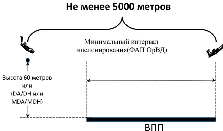
Рисунок 1. Горизонтальное эшелонирование операции «взлет–посадка»
