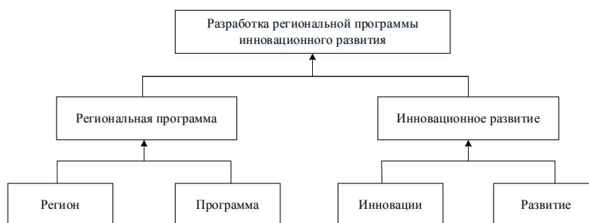
Рисунок 1. Терминологическая пирамида
